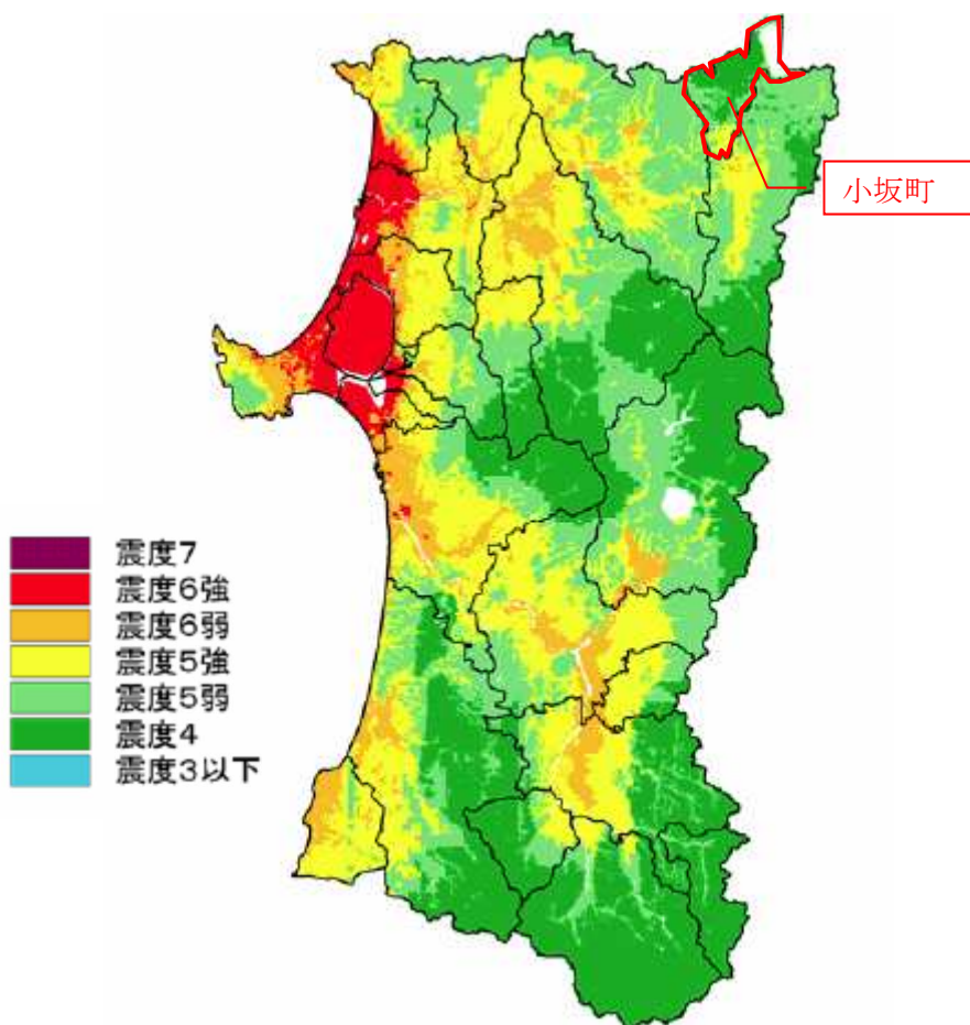
図2-1 想定海域A+B+C連動地震（M=8.7）による震度分布
