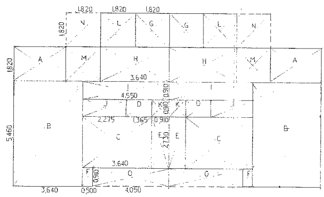
1階平面図 S=1:50
