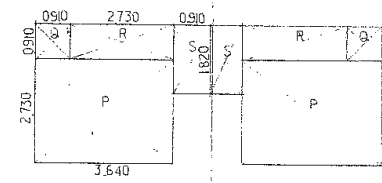
2階床構造図 S=1:100
