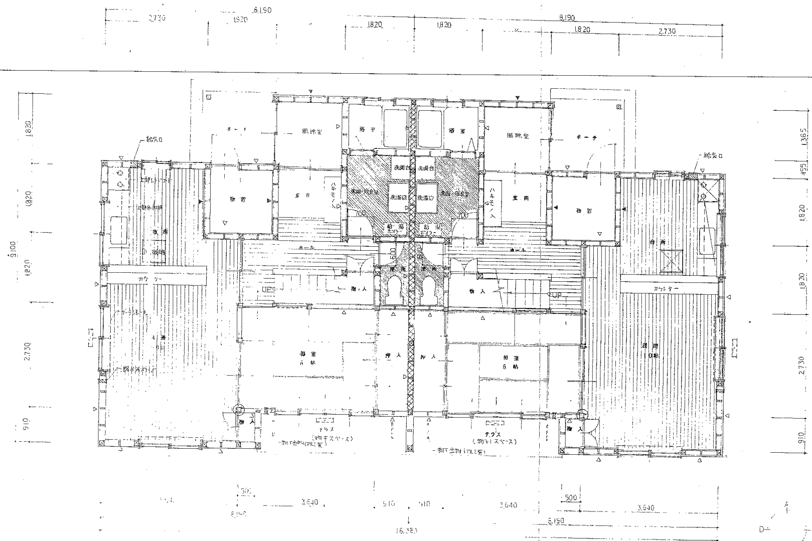
1階平面図 S = 1 : 50
