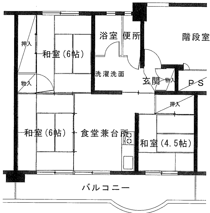
けやき宿舎標準間取り図
