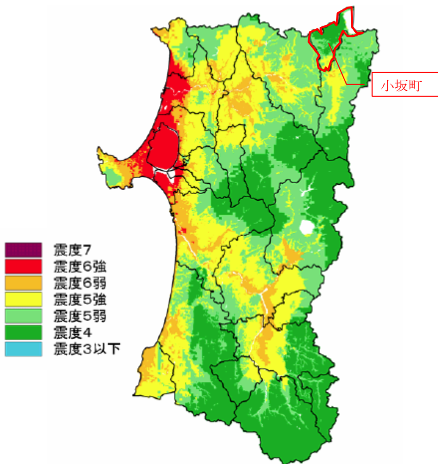
図 想定海域A+B+C連動地震（M=8.7）による震度分布
